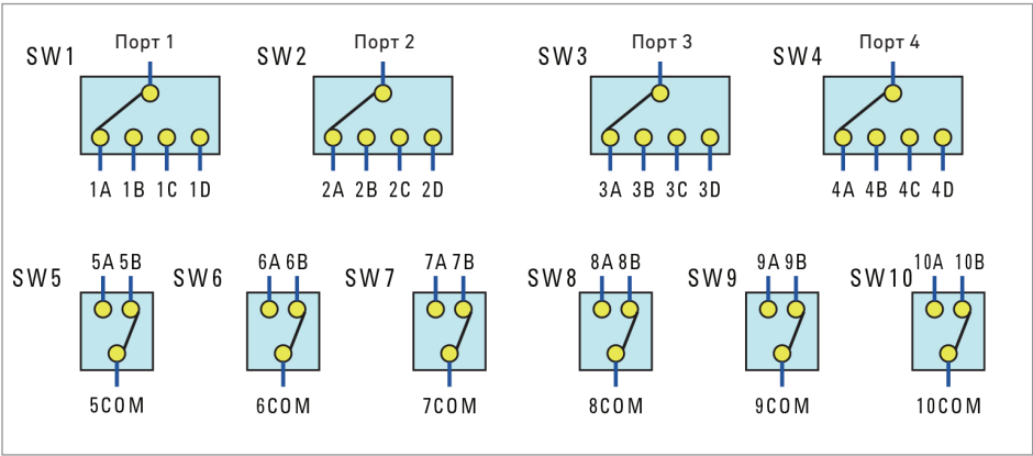
Рис. 14: Конфигурация коммутатора (E5092A-020)
