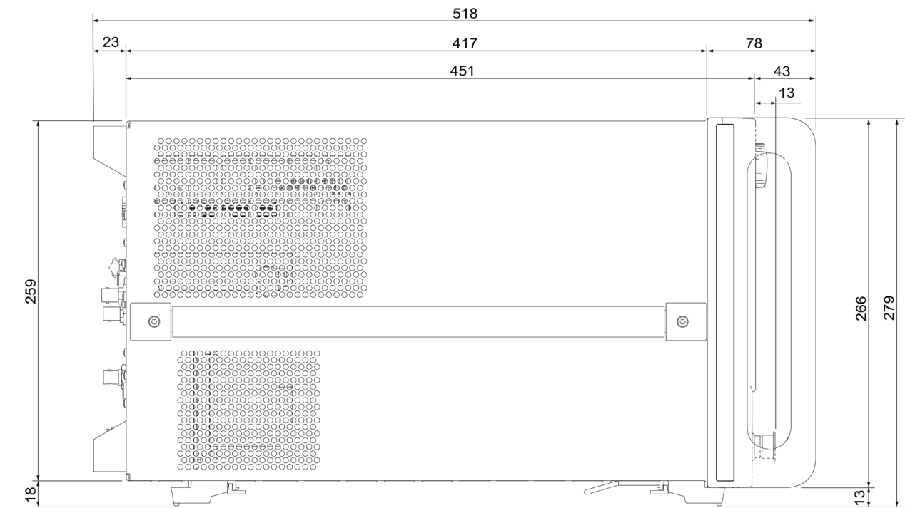
Размеры (вид сзади, опция 1E5, единица измерения – миллиметры)
